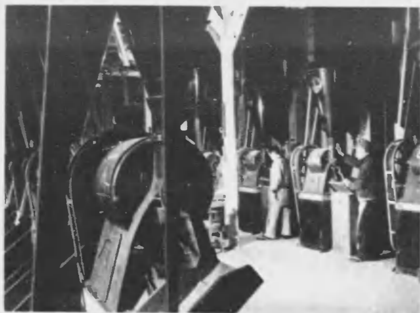
約一時間でお米十俵を呑む十量の精米機と、十五俵を呑む四臺の精米機を備へつけ、業者の企業合同精米所として日本一の稱ある愛知県米穀小賣商組合押切精米所の偉観
