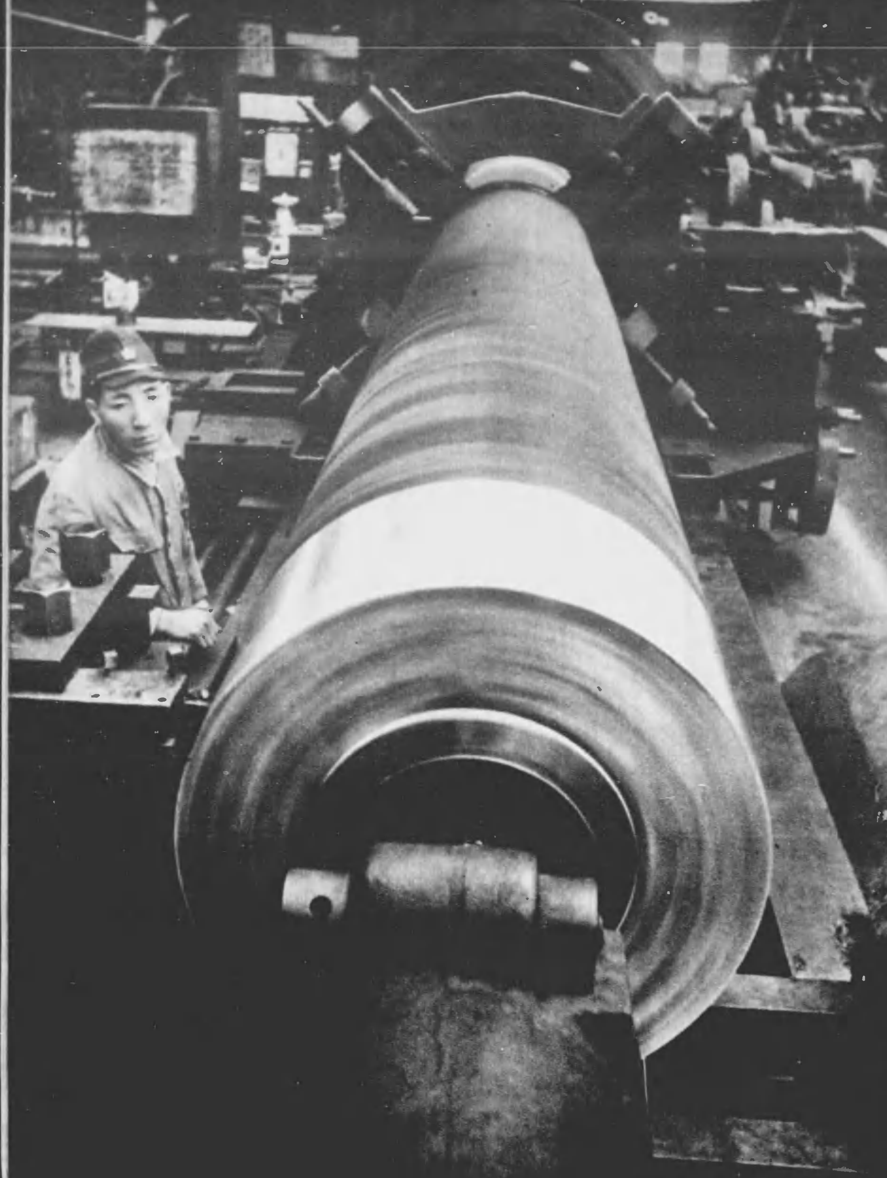
□ こんなすごい砲弾をうんと造つてもらはう——でき上つた重砲弾（陸軍兵器廠）
