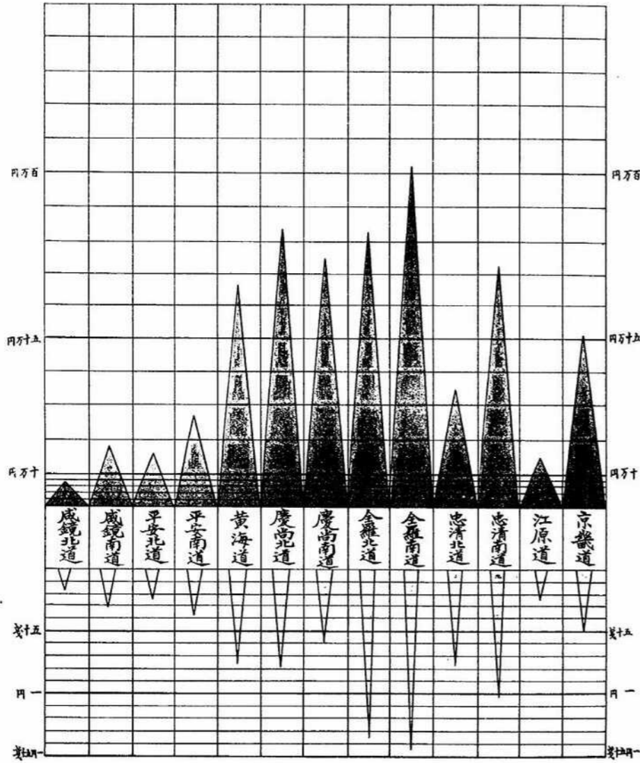
各道地稅課稅額比較(附人口一人負擔額)
