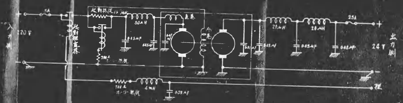
接続図
