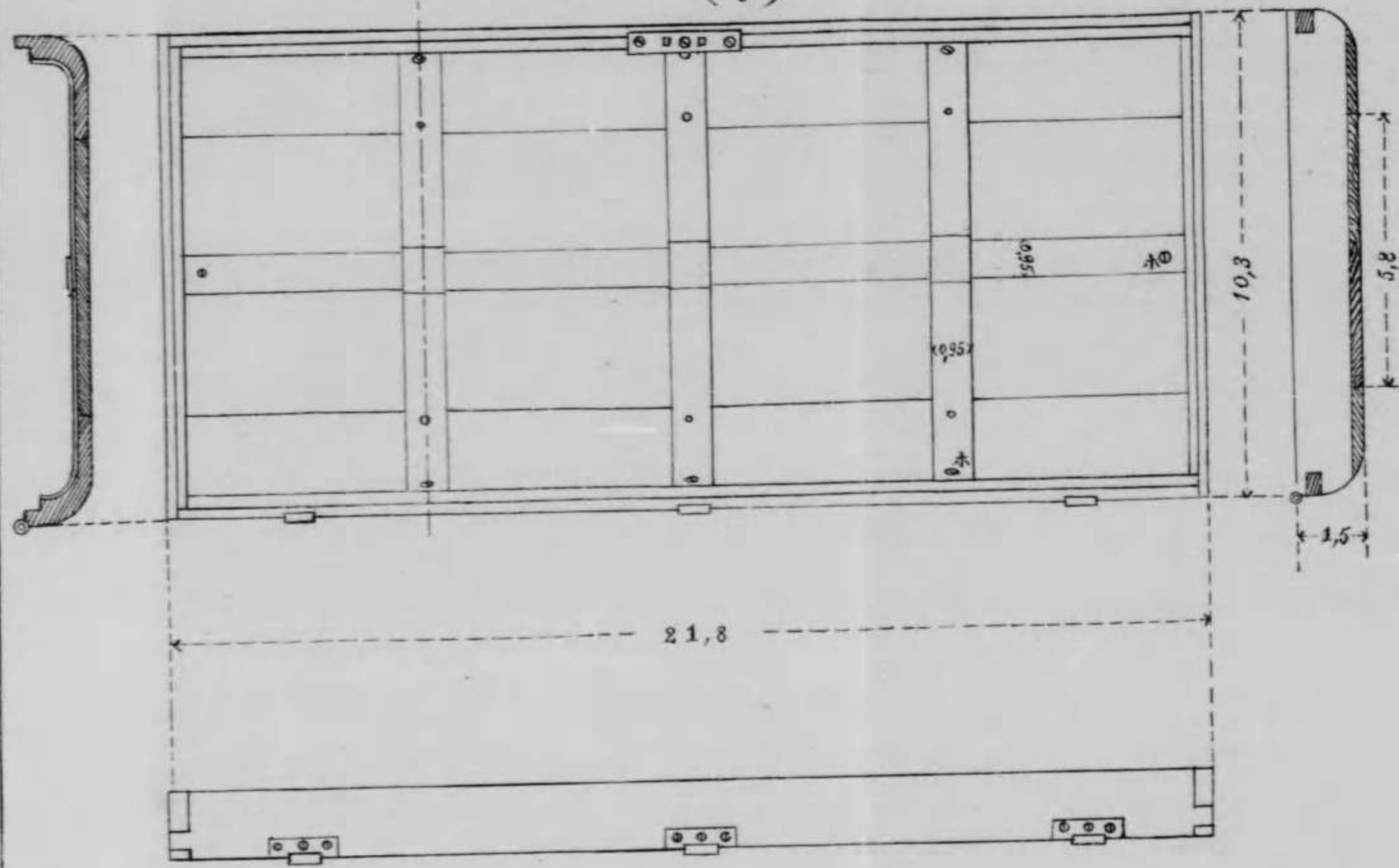
圖二十第 面內蓋 ( \frac{1}{5} )
