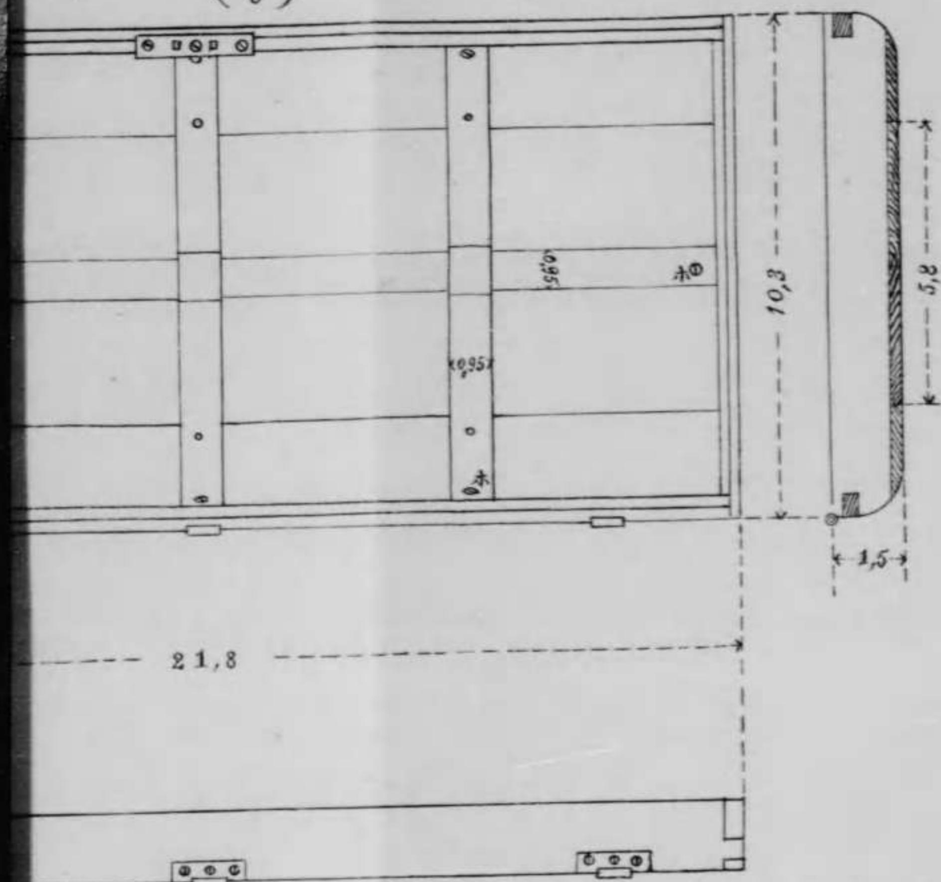
圖二十第 內蓋 ( \frac{1}{5} )
