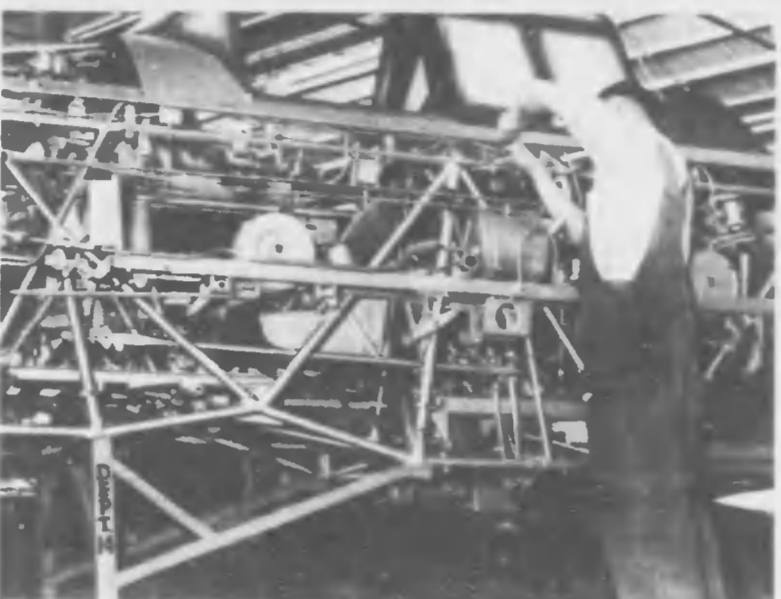
組立作業中のウイラウエイ機の胴體部
