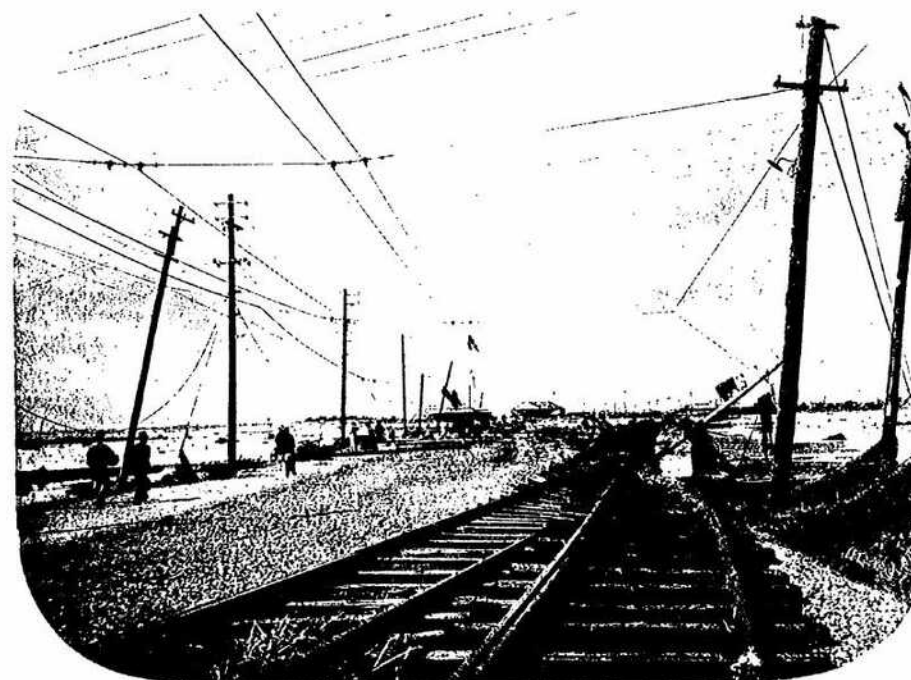
堺市阪堺電鐵會社出島海岸線路ノ被害
