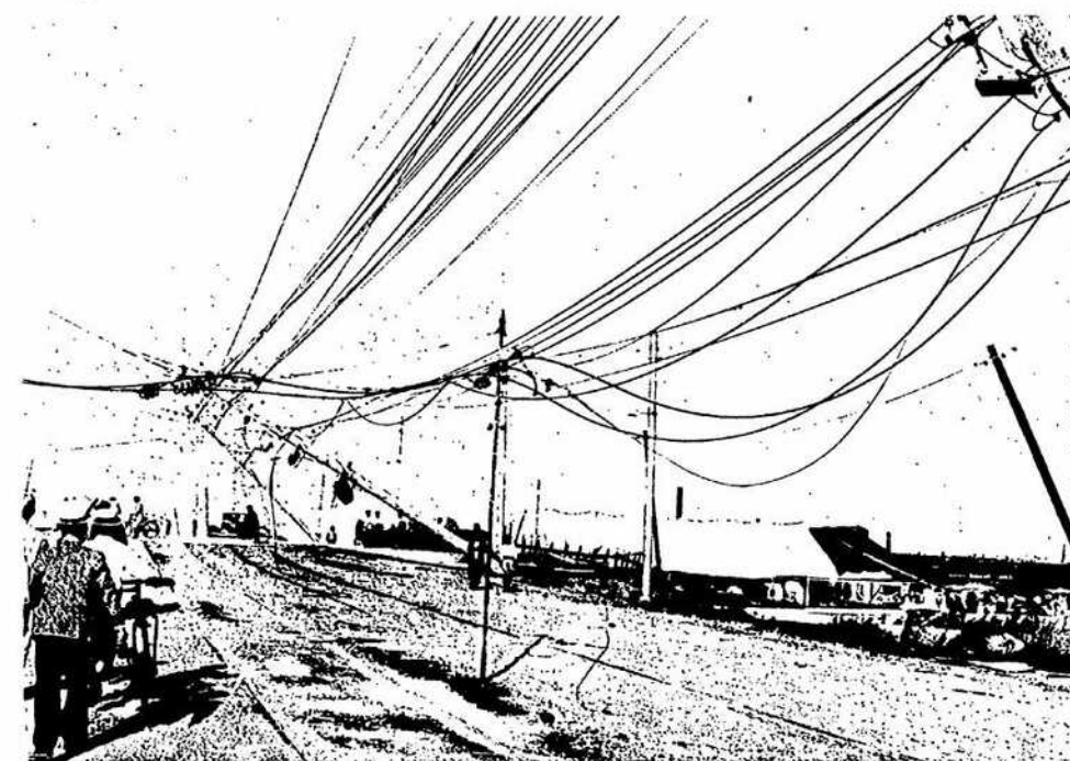
大阪市内此花區春日出櫻島間ノ電柱 電線ノ被害 同附近一帯一時ハ一面ノ海ト化ス
