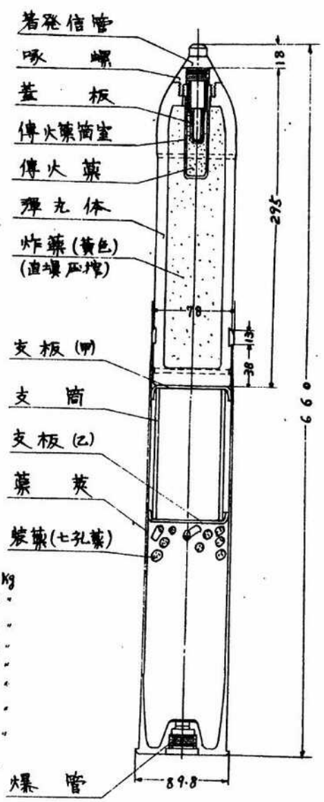
乙式榴彈藥筒(甲)
