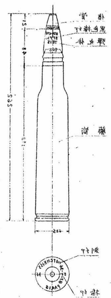
榴彈彈藥筒
